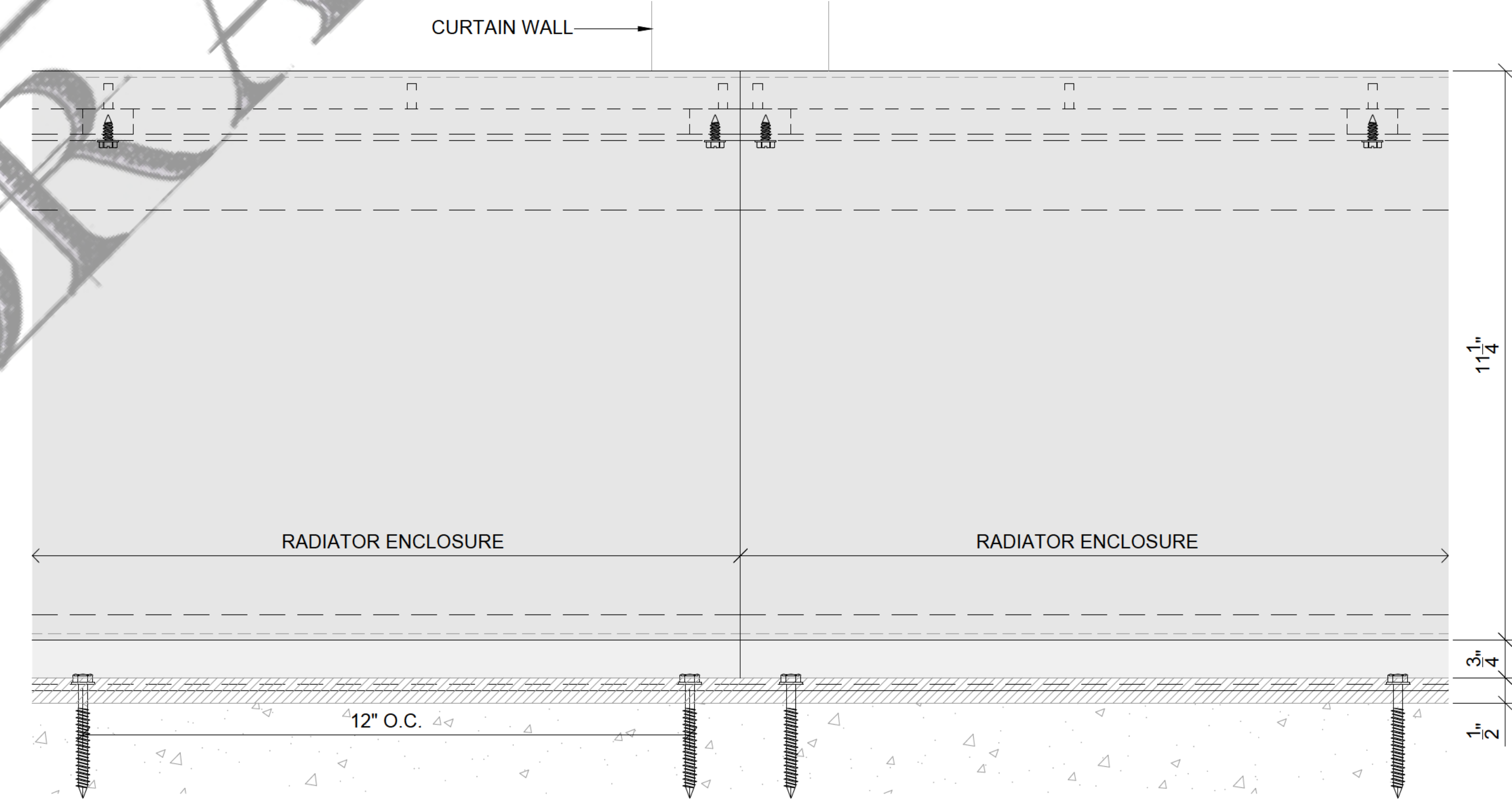
3E-1 ELEVATION
